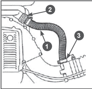
Рис. 12 Установка шланга распылителя
