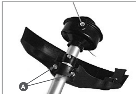
Рис. 2 Установка защитного кожуха
